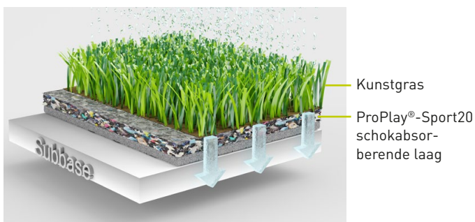
Kunstgrassysteem met ProPlay ® -Sport schokabsorberende laag
