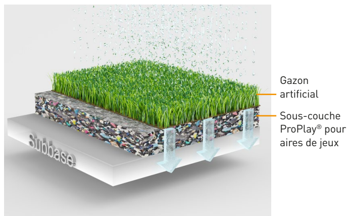
Système de gazon artificiel avec ProPlay® pour aires de jeux avec sous-couche de protection contre les chutes
